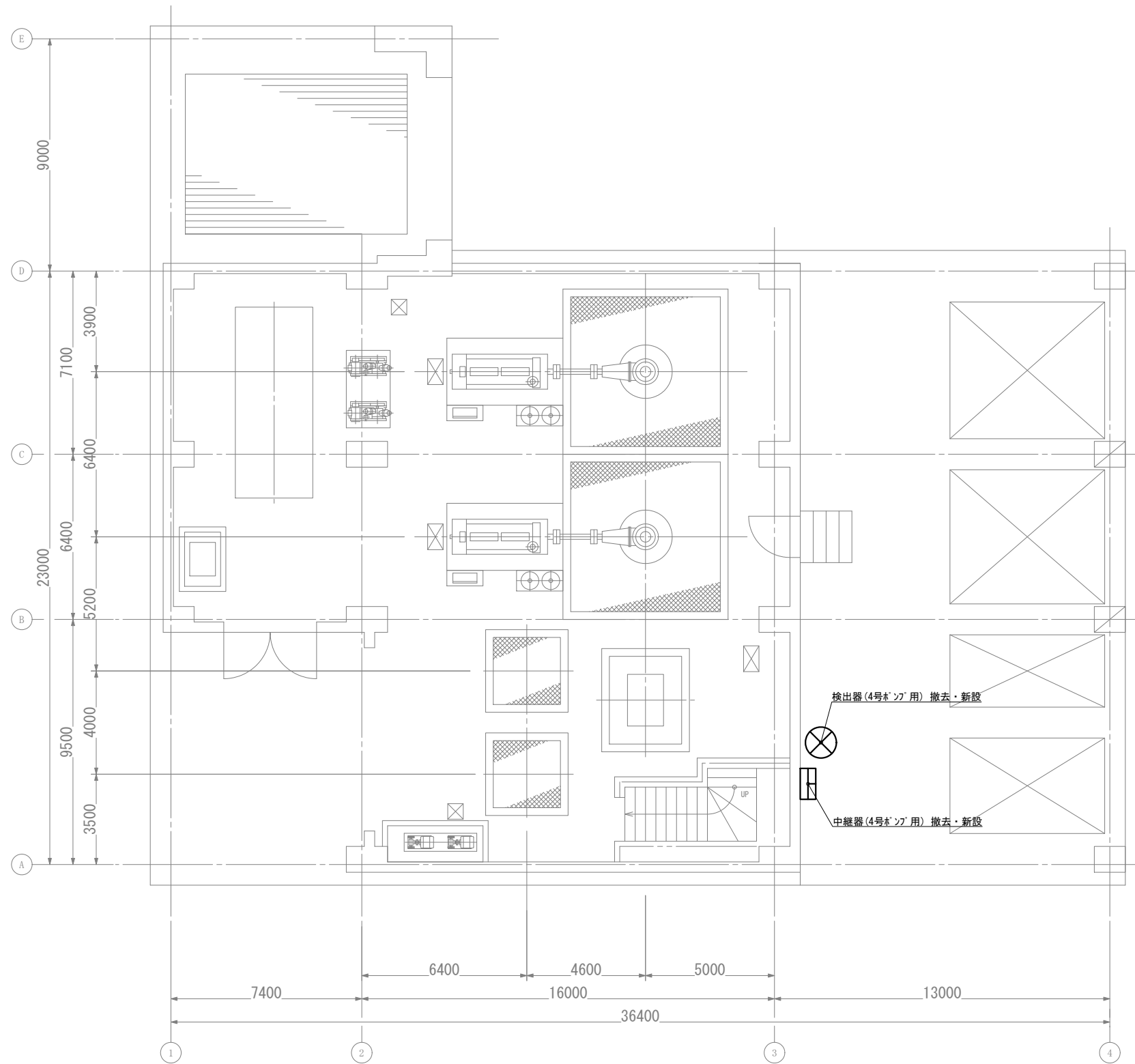
1階平面図 (A3:1/200)
