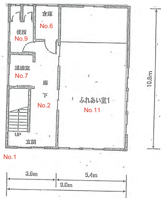
1 階
