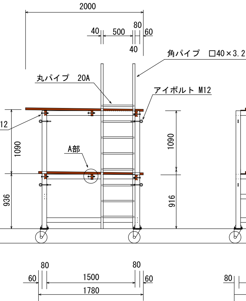
側面図
