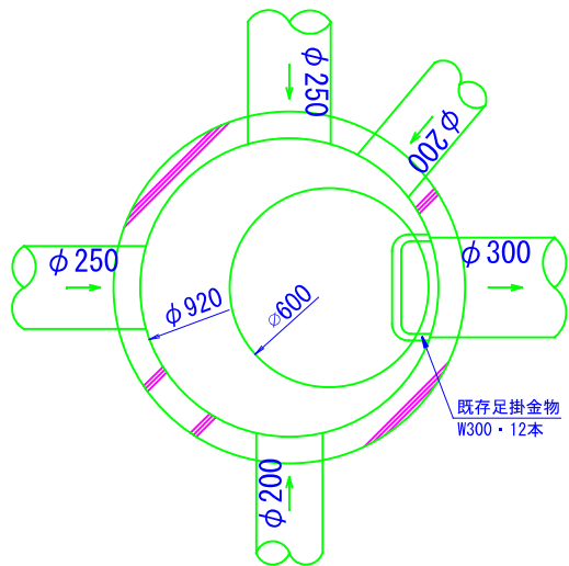
現状図 平面図
