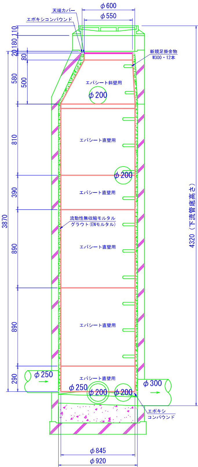
提案図 断面図
