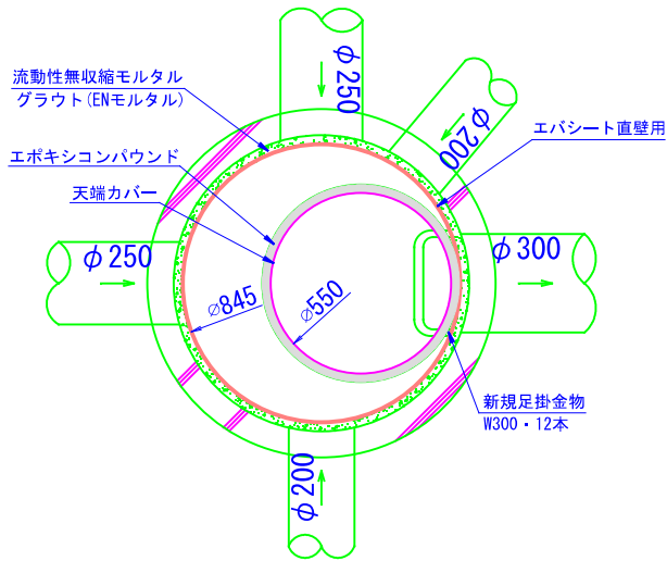
提案図 平面図
