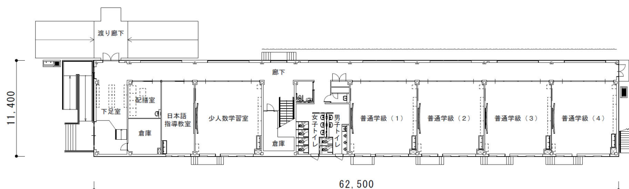
1階平面図
