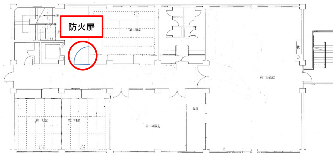
3階平面図 S:1/100
