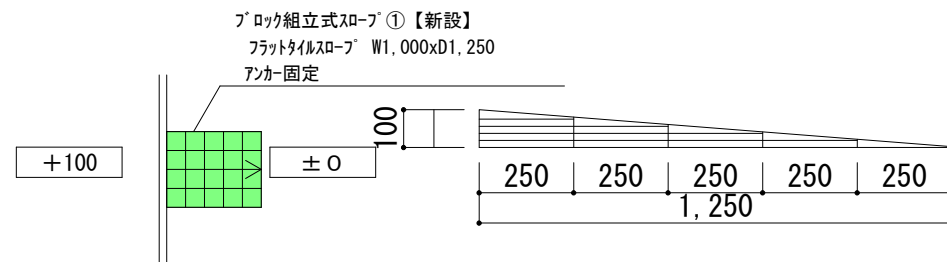
改修後平面図 S=1/100
