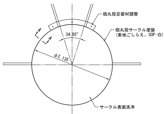
平 面 図
