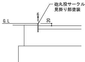
A-A断面図 S=1:10
