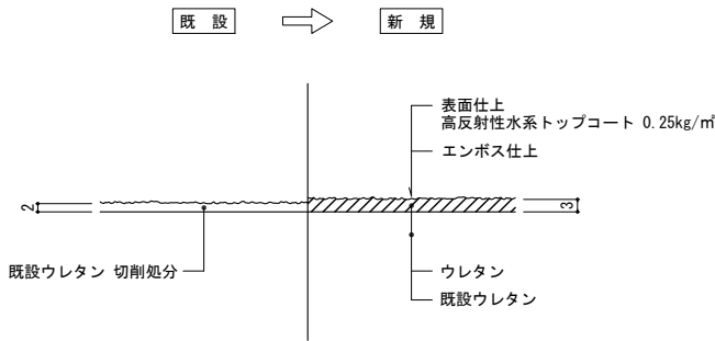
ウレタン切削オーバーレイ 詳細図 S=1:1
