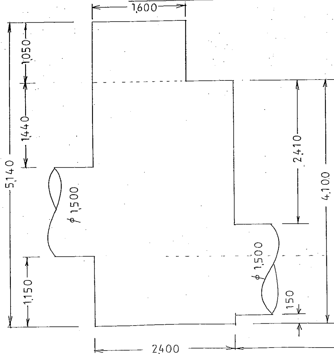
断面図
