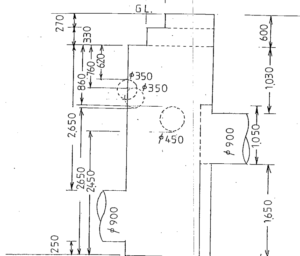
断面図 s \frac{1}{400}
