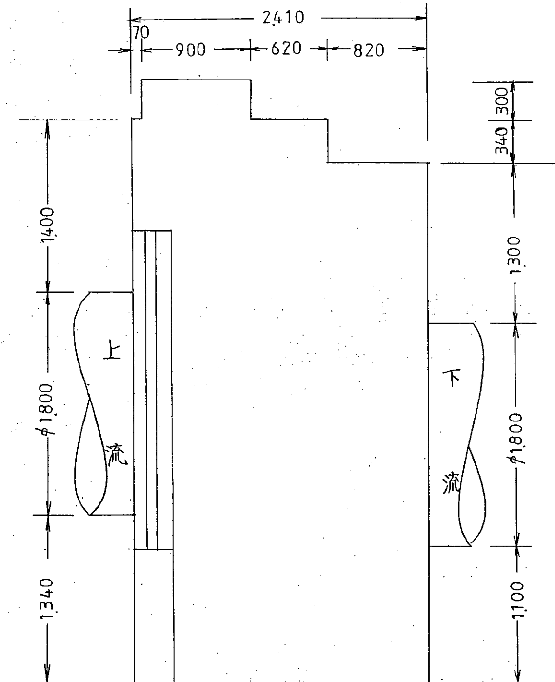
NO.2 断面図 s \frac{1}{300}
