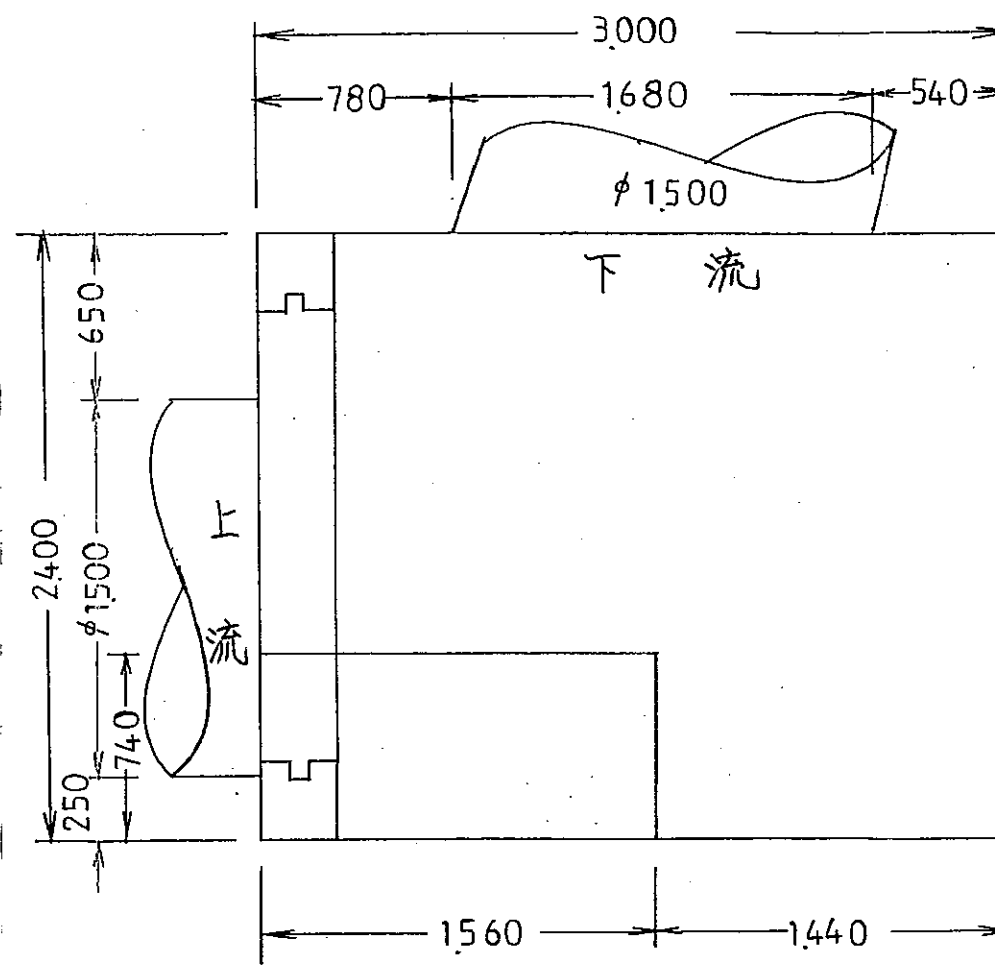
NO.3 平面図 s \frac{1}{300}
