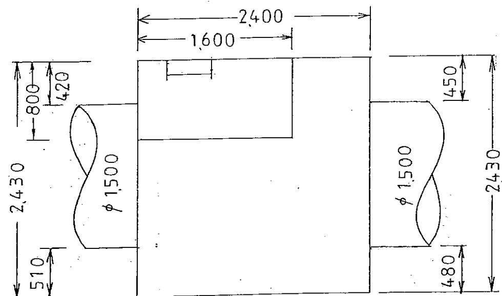
断面図
