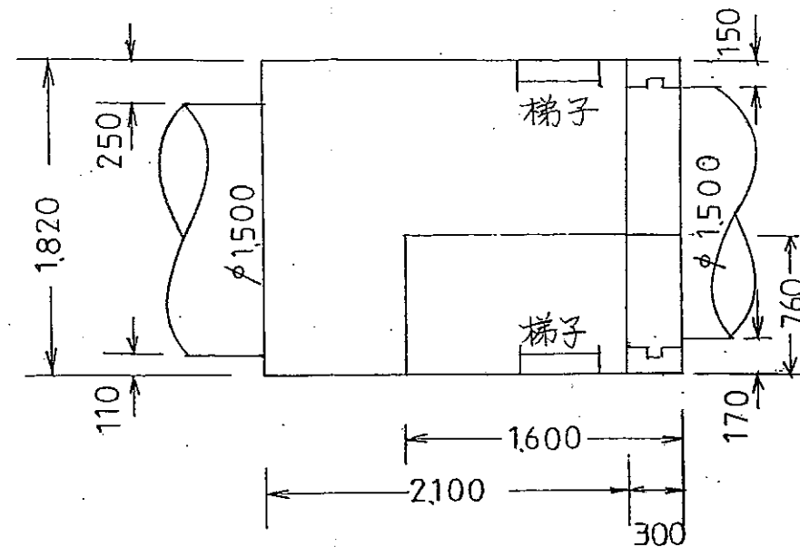
GL 断面図
