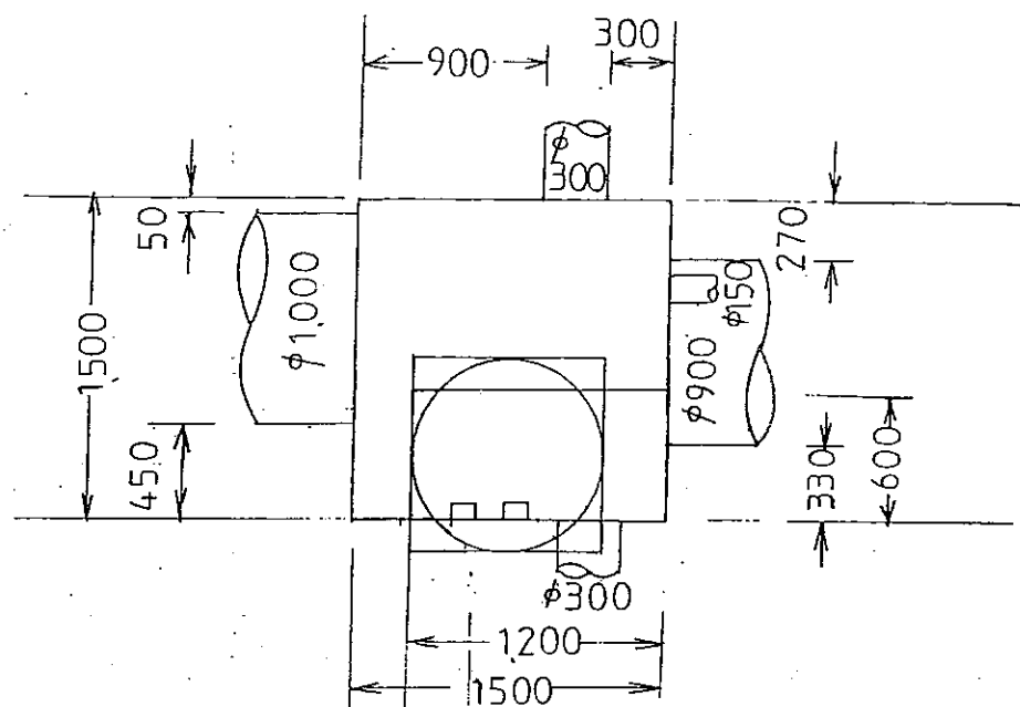
No.2 下流平面図 s \frac{1}{400}
