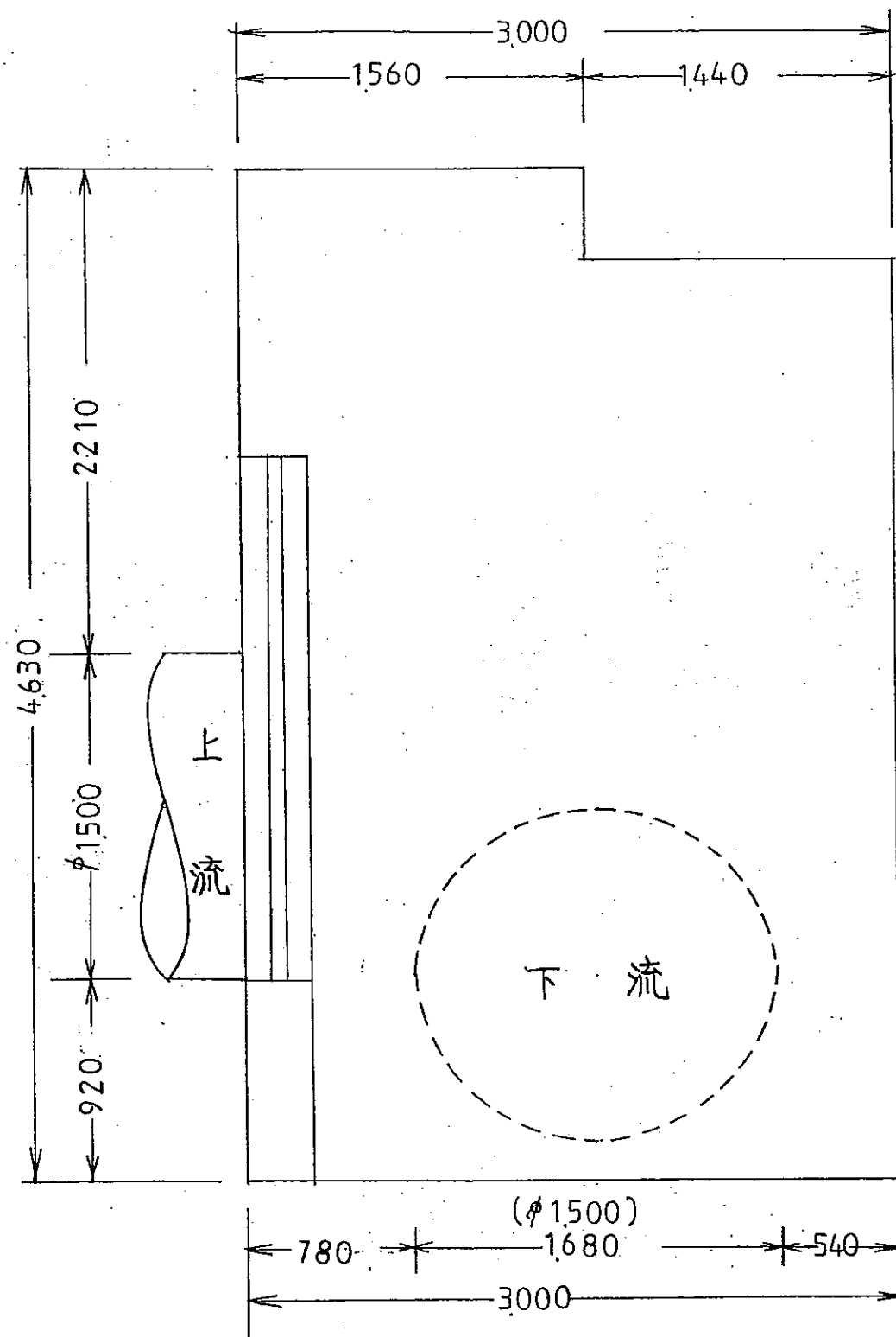
NO.3 断面図 s \frac{1}{300}
