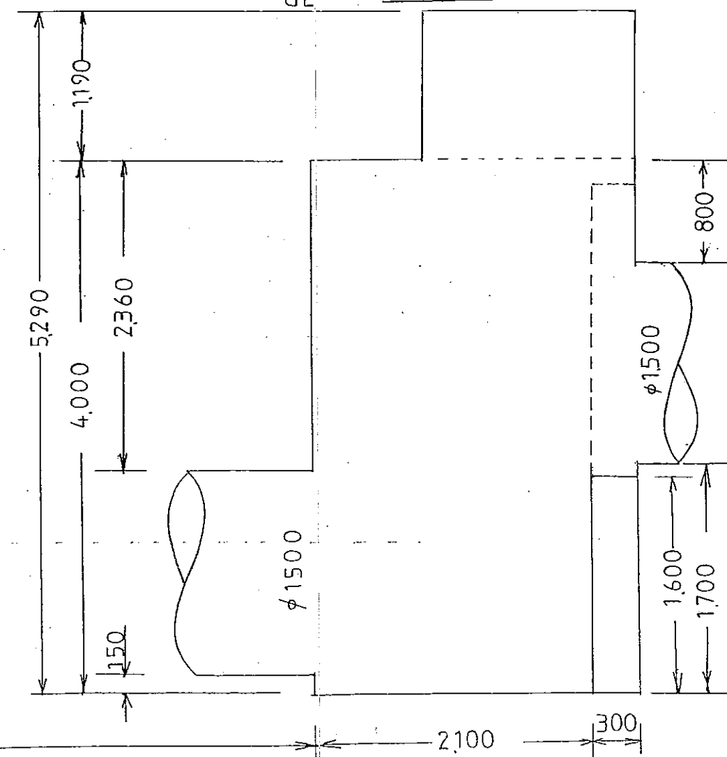
断面図
