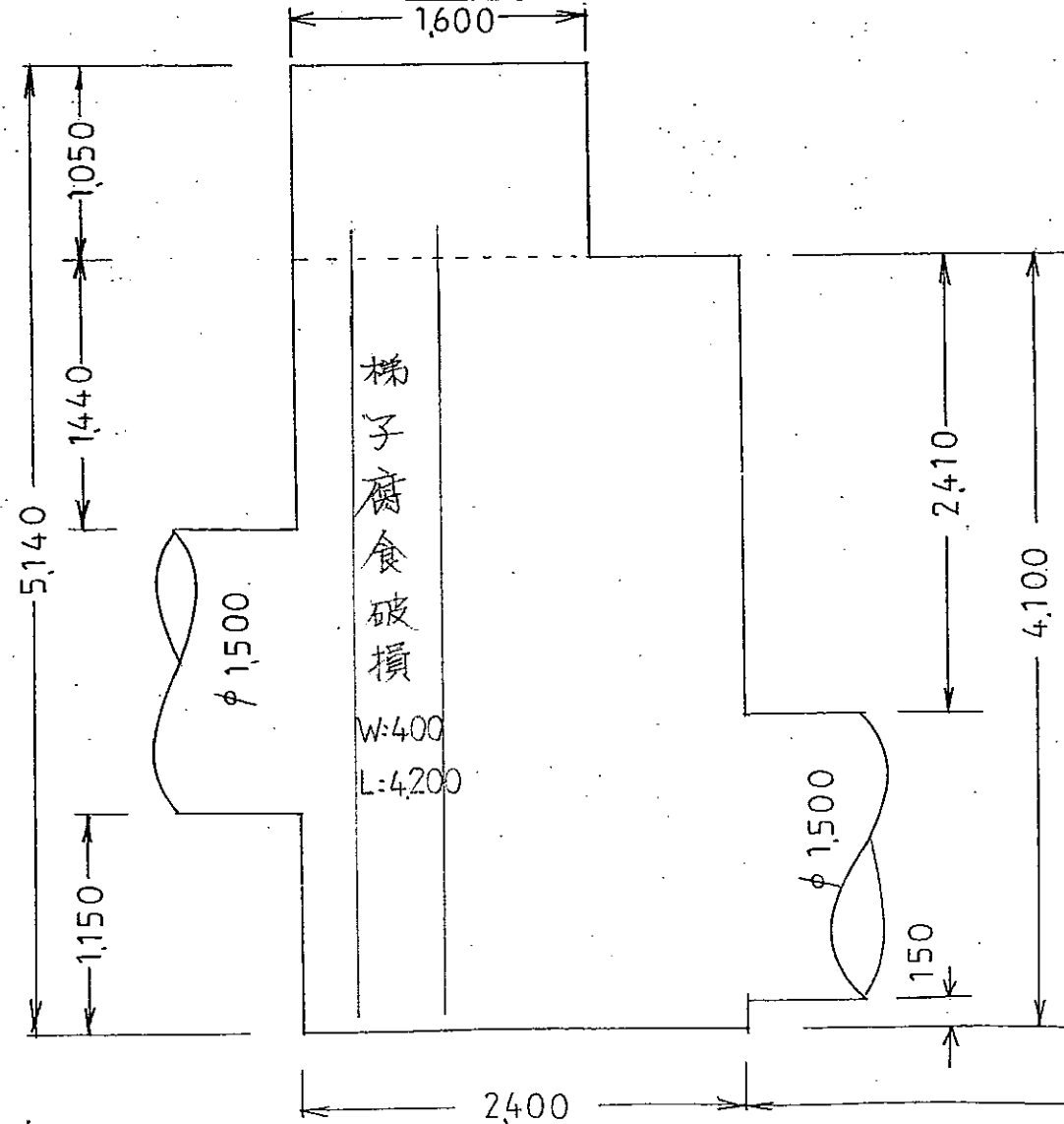
断面図
