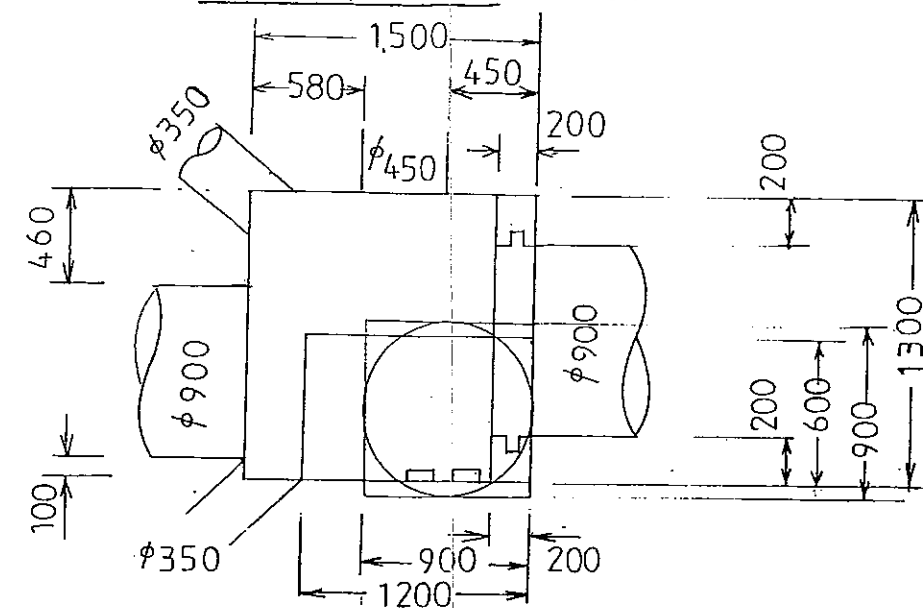
No.1 上流平面図 s \frac{1}{400}
