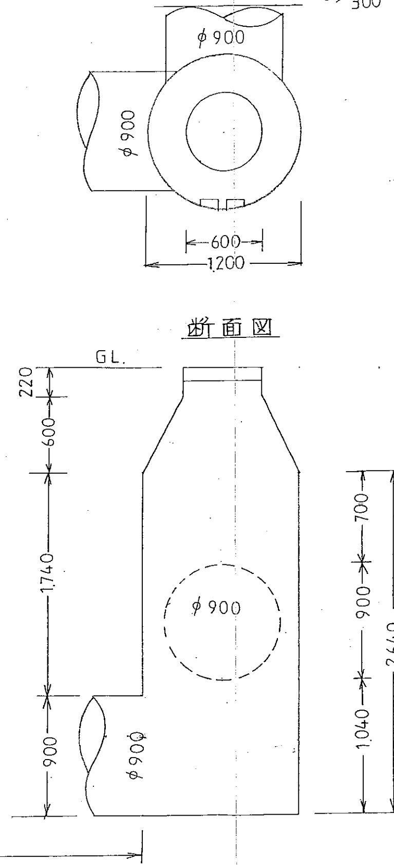
No.2 下流平面図 s \frac{1}{300}
