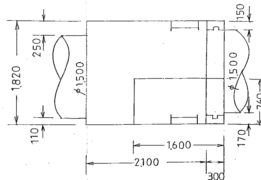
断面図
