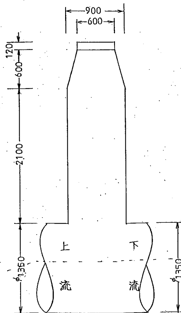
断面図 \frac{1}{300}
