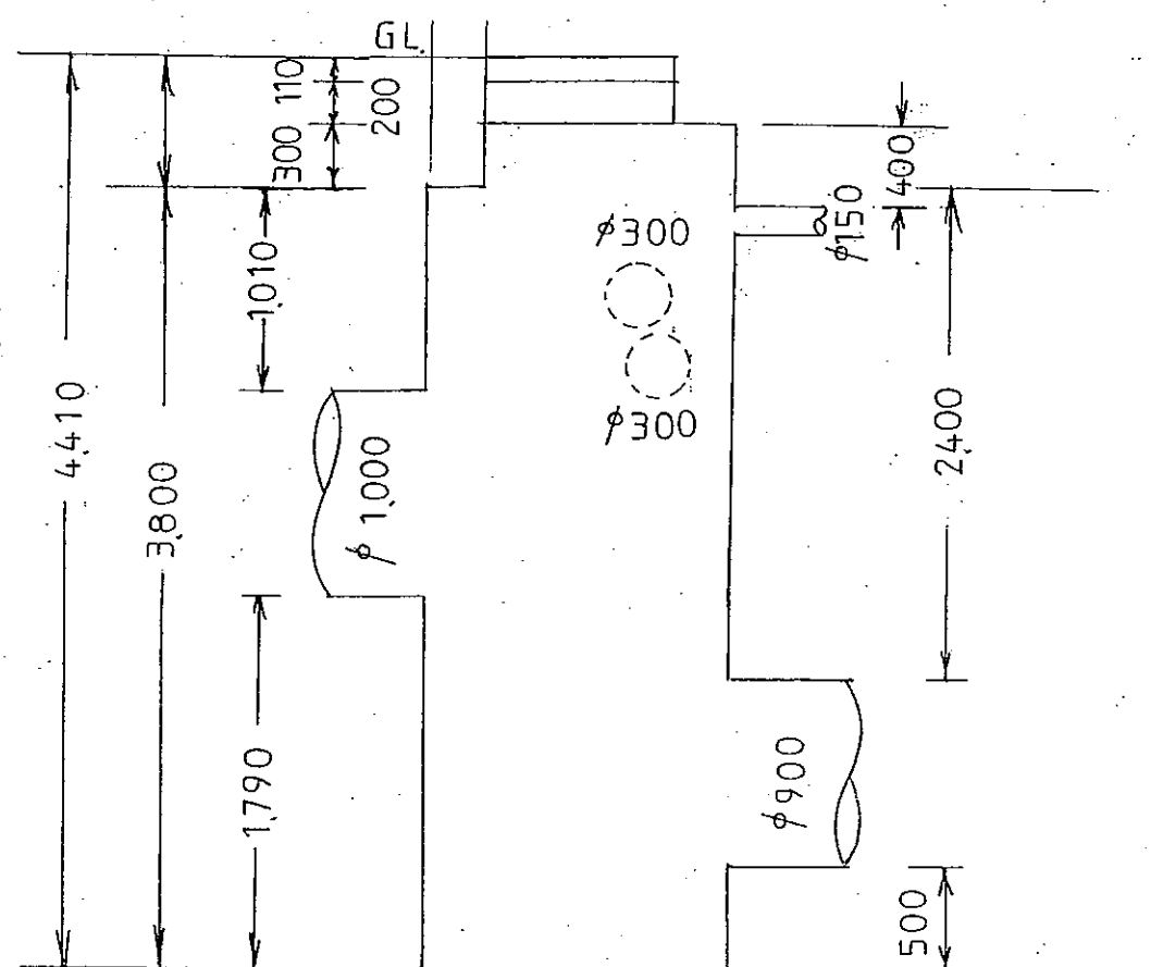
断面図 s \frac{1}{400}
