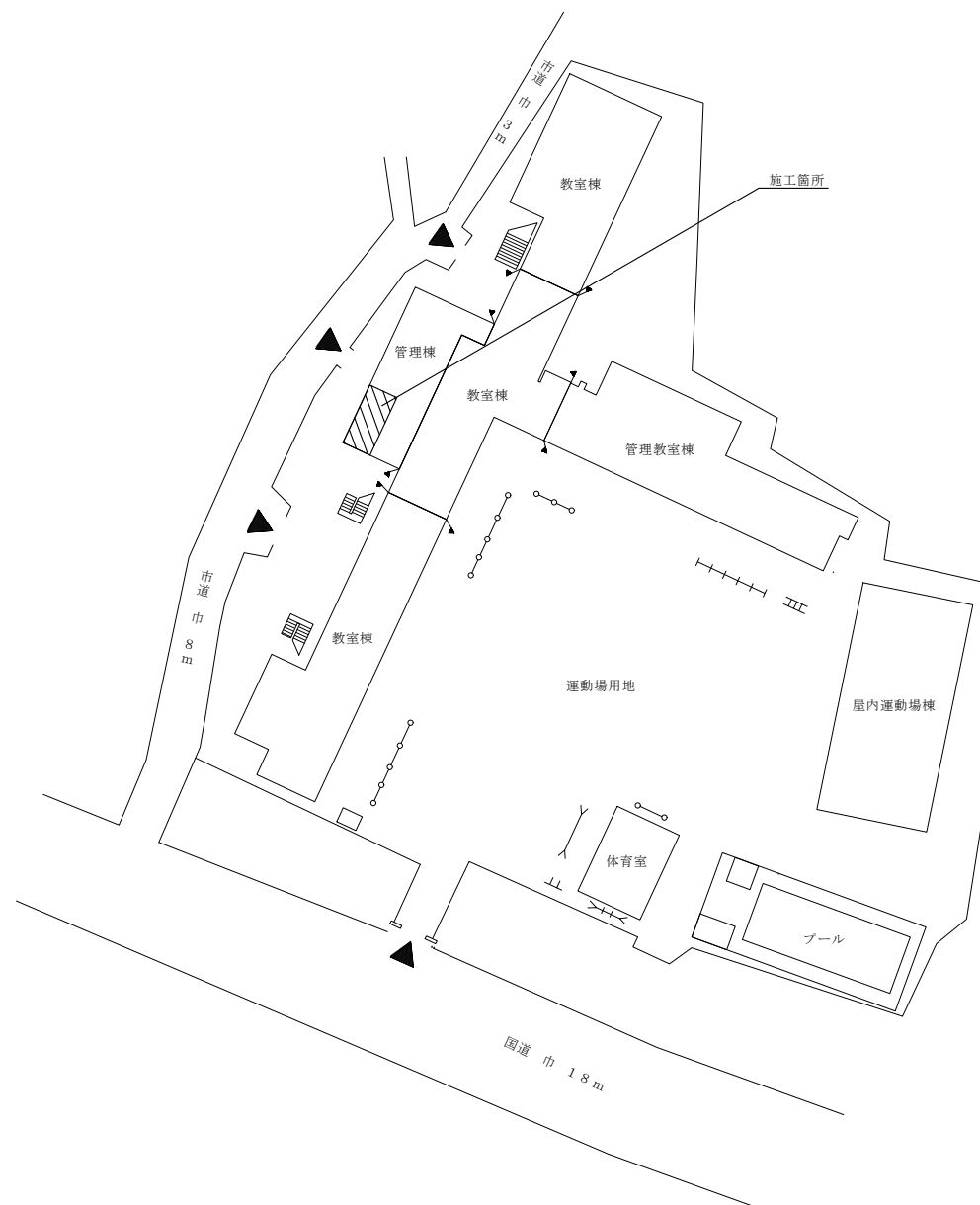
配置図 S=1/1200
