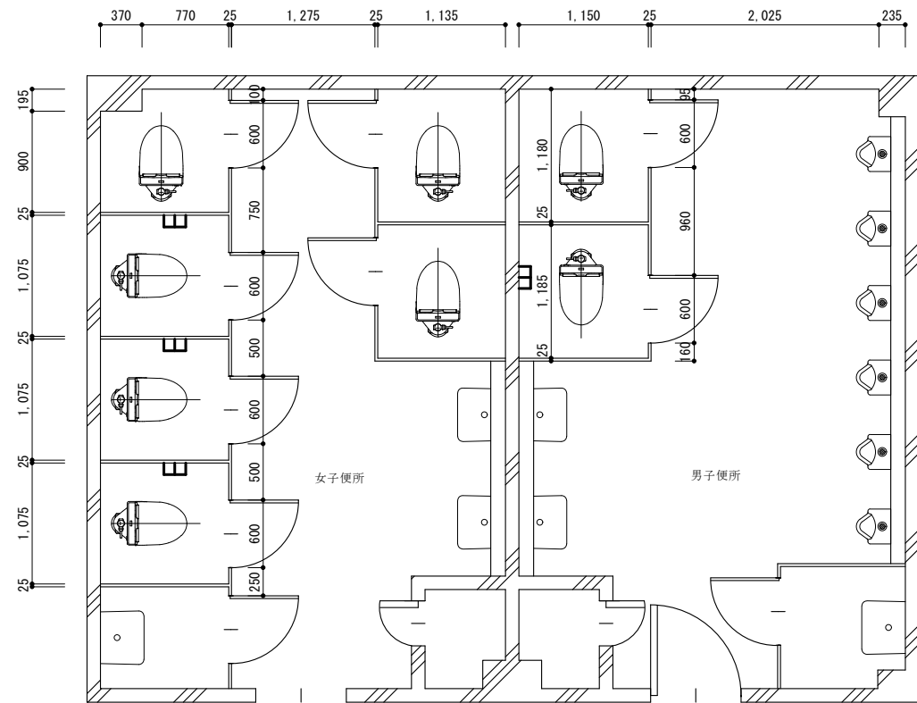
【改修】2棟北側2階～3階便所平面詳細図 S=1/60
