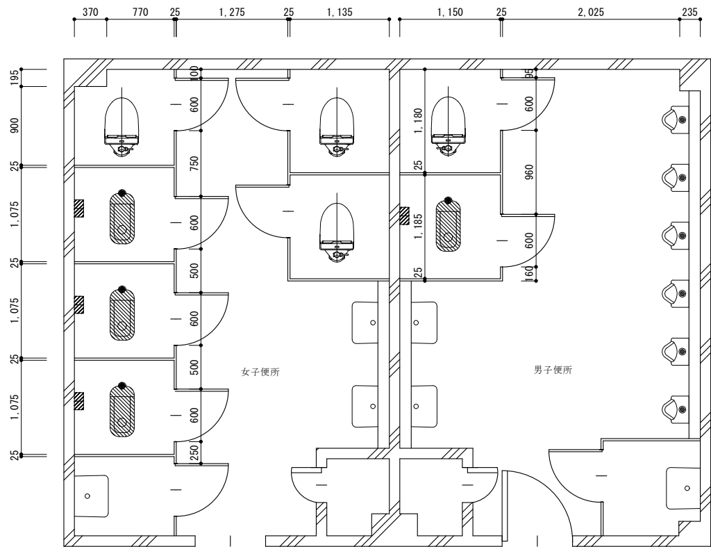
【既存】2棟北側2階～3階便所平面詳細図 S=1/60
