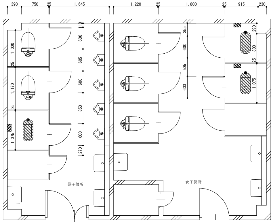
【既存】2棟北側1階便所平面詳細図 S=1/60
