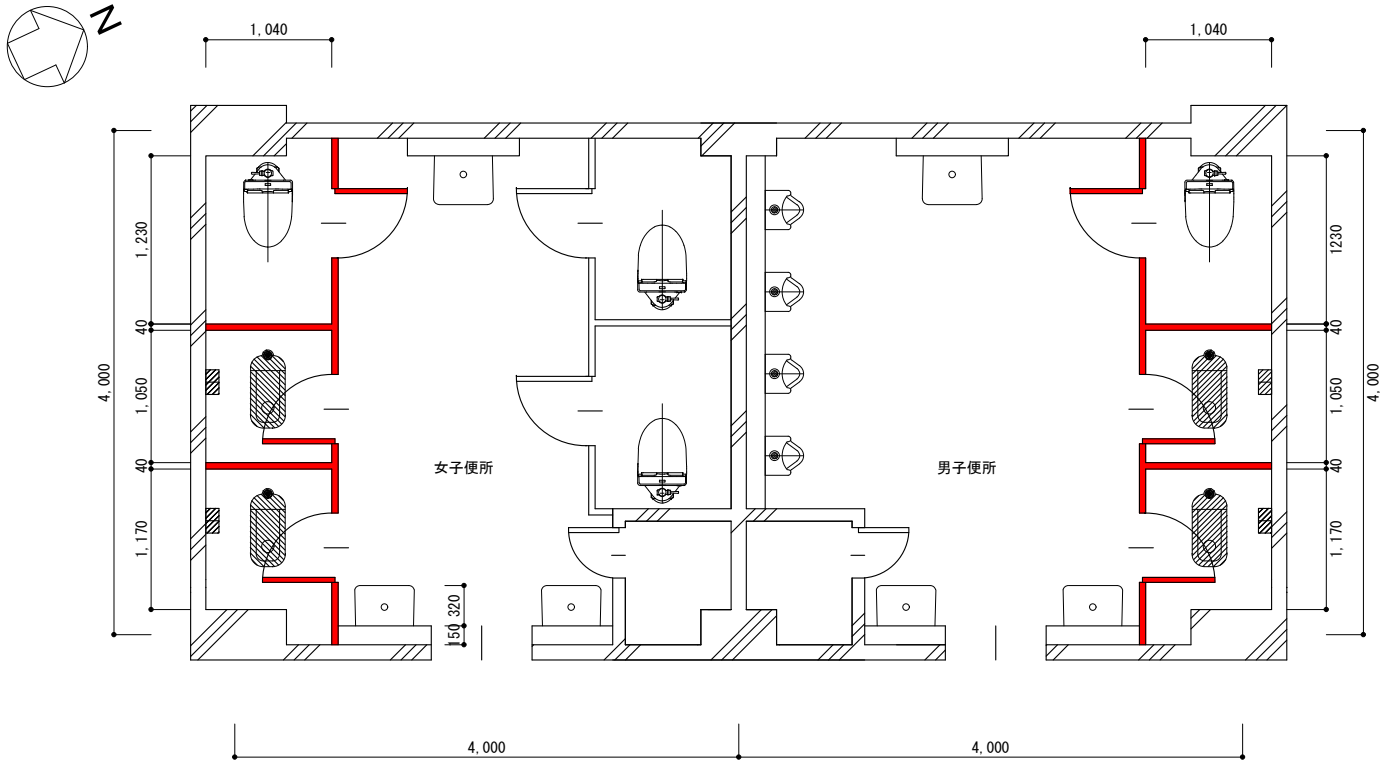
【既存】1-3棟1～3階便所平面詳細図 S=1/60
