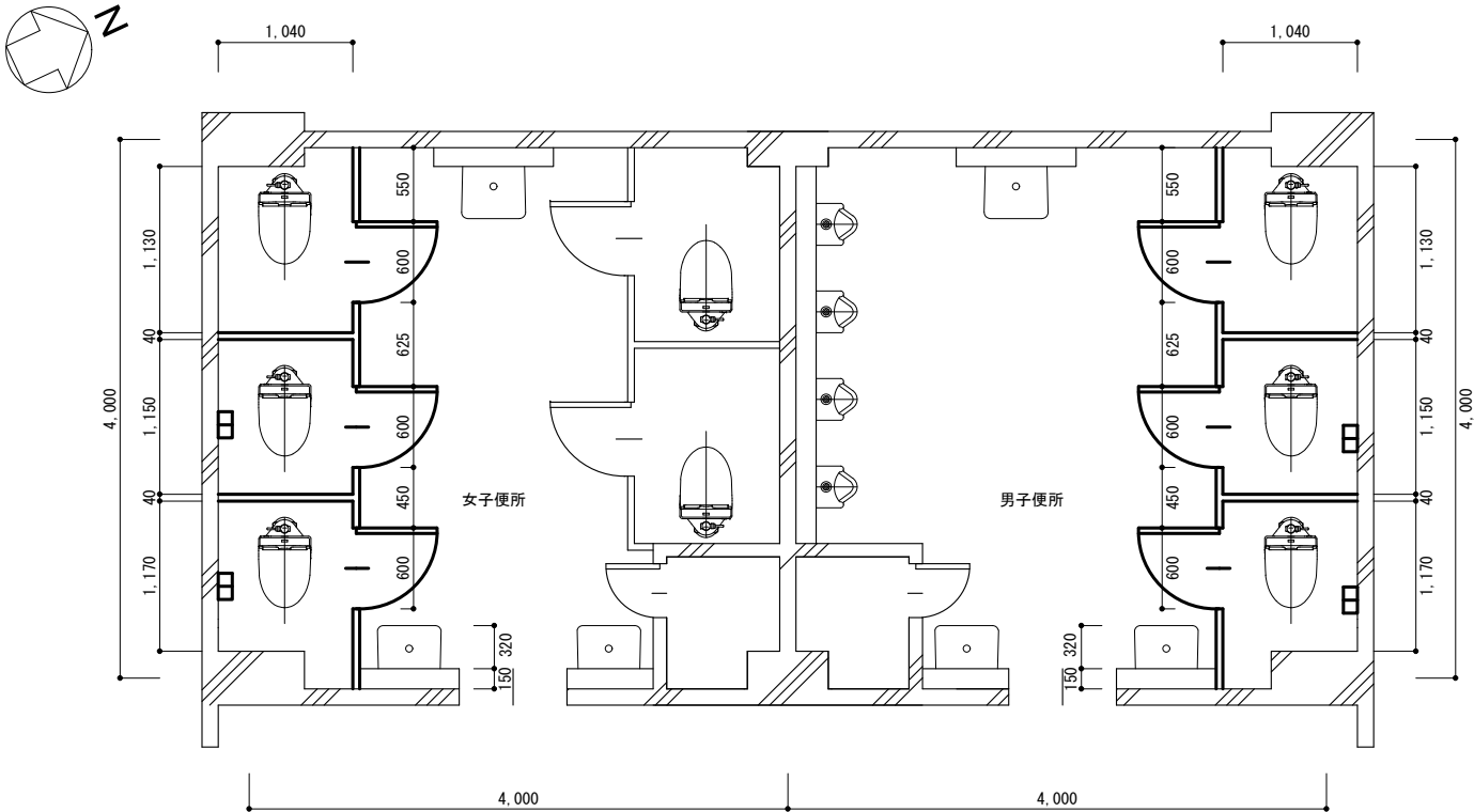
【改修】1-3棟1～3階便所平面詳細図 S=1/60
